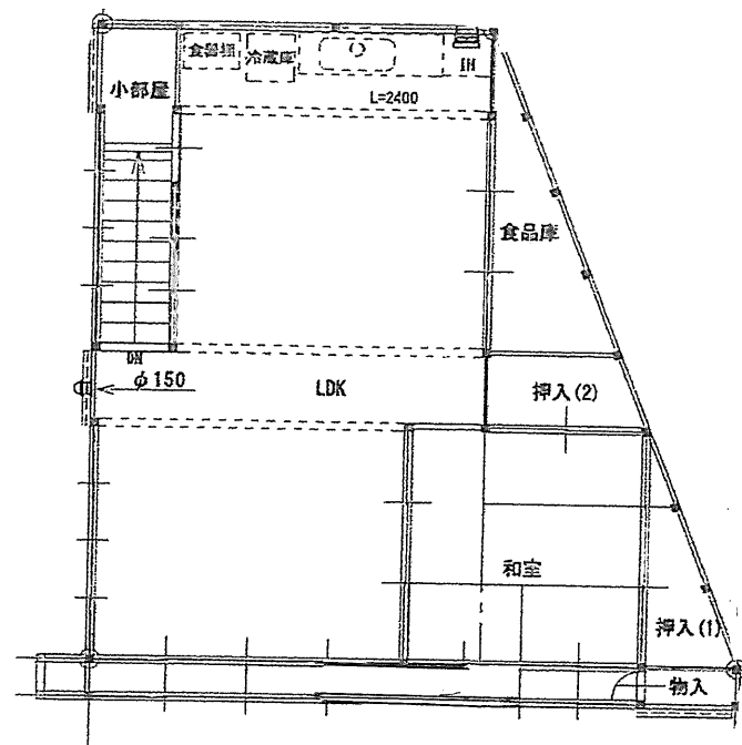
2階平面図
